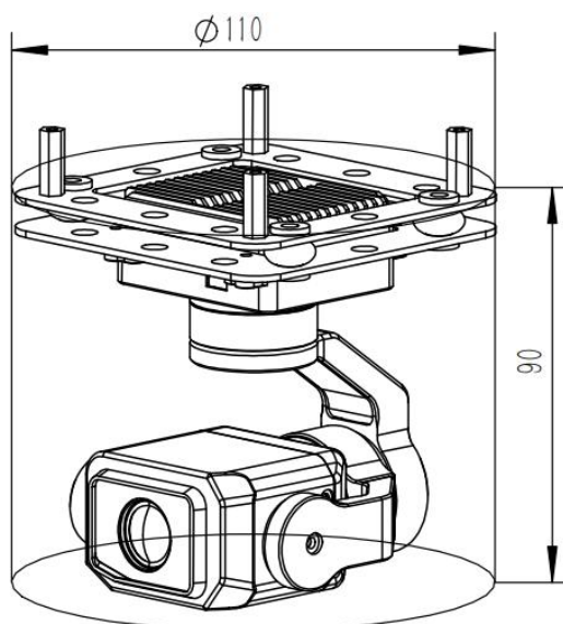
图 1-1-1 单光一体云台结构
