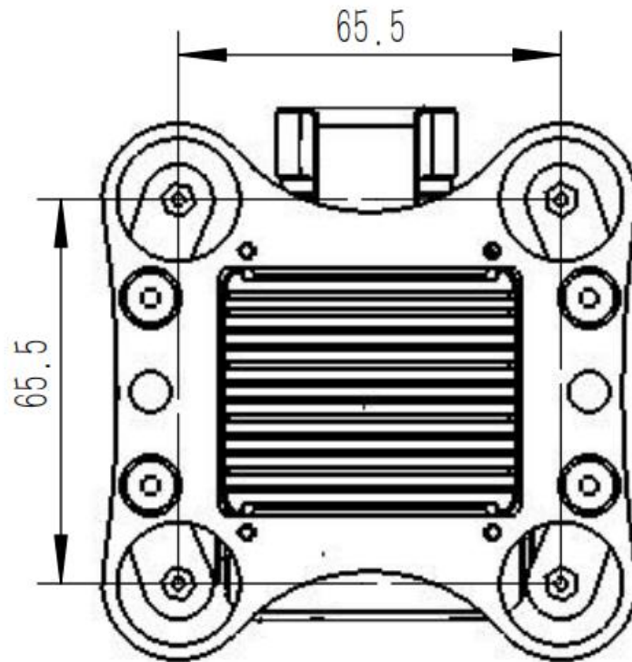
图 3-1-1：双光云台对外机械接口
