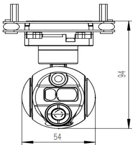
图 1-1-1 三光一体云台结构
