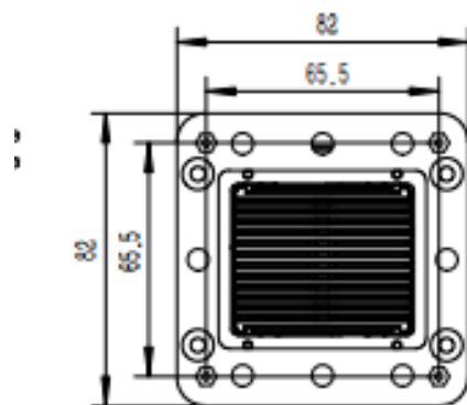
图 3-1-1: 双光云台对外机械接口
