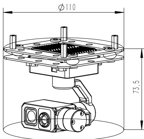
图 1-1-1 双光一体云台结构
