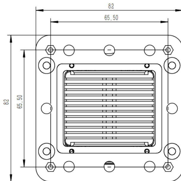
图 3-1-1：双光云台对外机械接口
