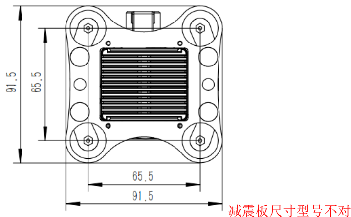
图 3-1-1: 双光云台对外机械接口
