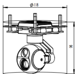
图 1-1-1 双光一体云台结构
