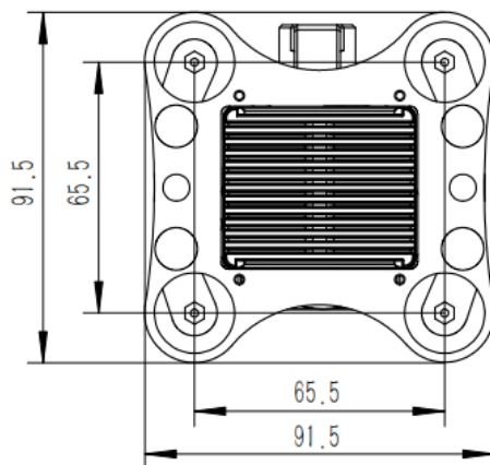
图 3-1-1: 双光云台对外机械接口
