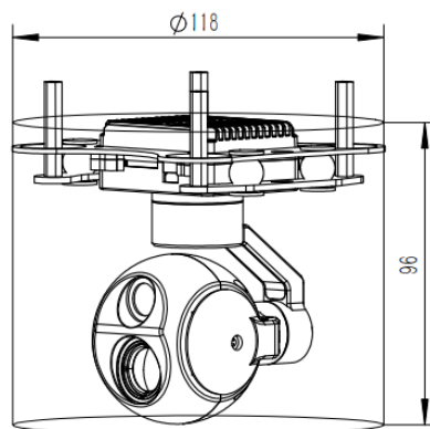
图 1-1-1 双光一体云台结构
