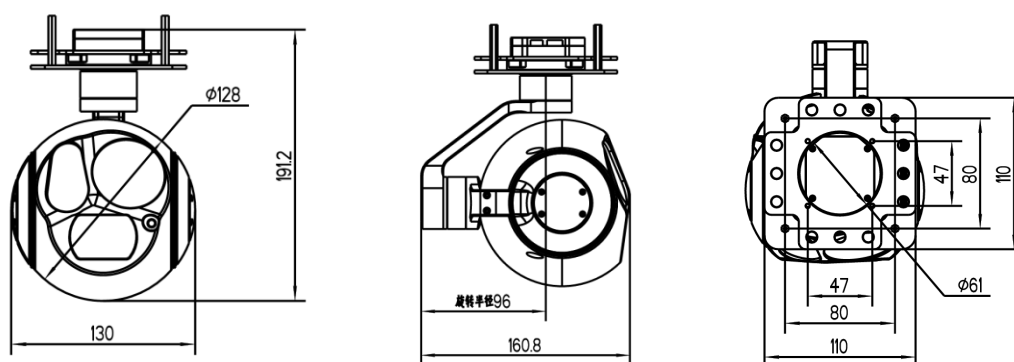
图 1-1-1 三光一体云台结构
