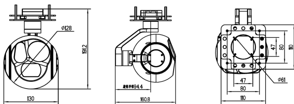
图 1-1-1 三光一体云台结构
