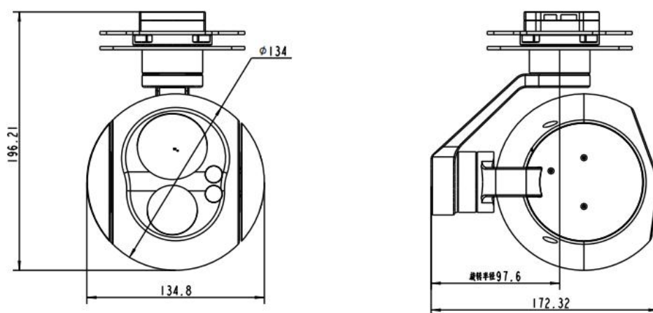
图 1-1-1 三光一体云台结构
