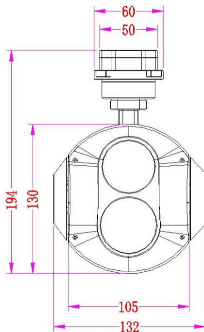
图 1-1-1 双光一体云台结构
