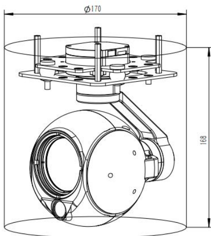
图 1-1-1 双光一体云台结构
