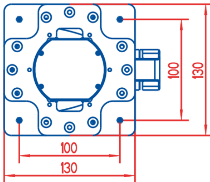
图 3-1-1：双光云台对外机械接口
