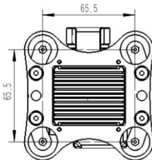
图 3-1-1：单光云台对外机械接口
