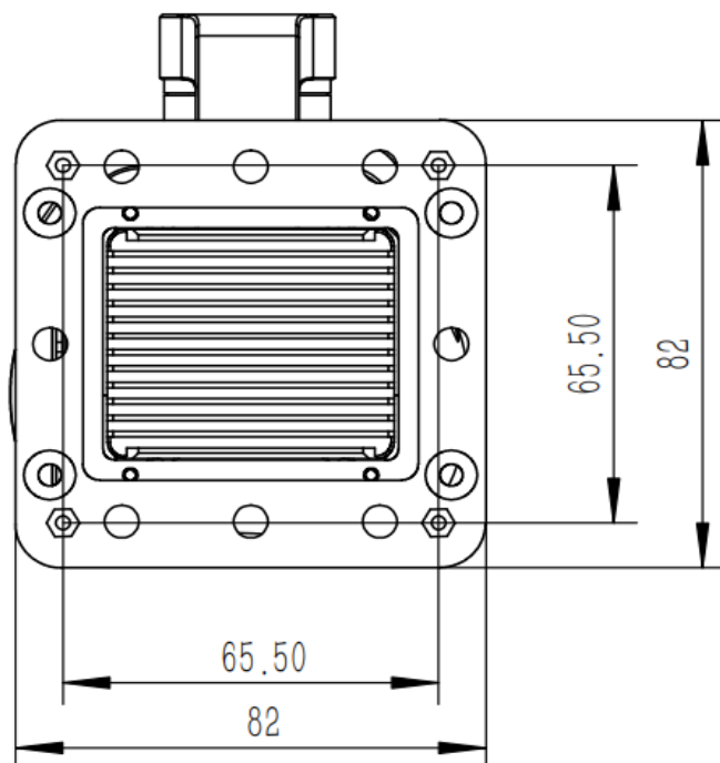
图 3-1-1：双光云台对外机械接口
