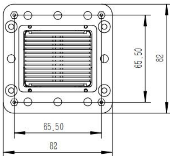
图 3-1-1：单光云台对外机械接口
