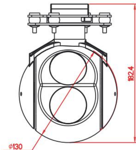
图 1-1-1 双光一体云台结构
