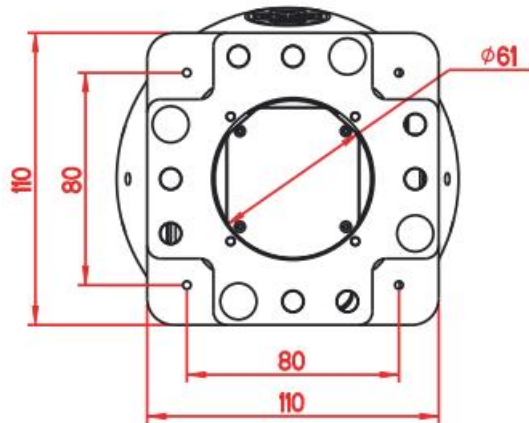
图 3-1-1：双光云台对外机械接口
