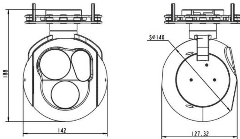
图 1-1-1 双光一体云台结构
