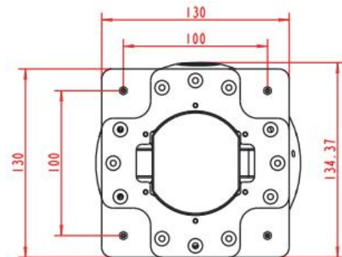
图 3-1-1：双光云台对外机械接口
