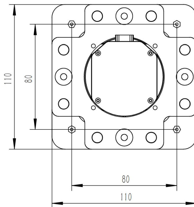
图 3-1-1：三光云台对外机械接口
