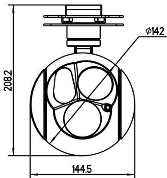
图 1-1-1 四光一体云台结构
