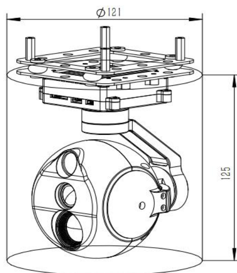
图 1-1-1 三光一体云台结构
