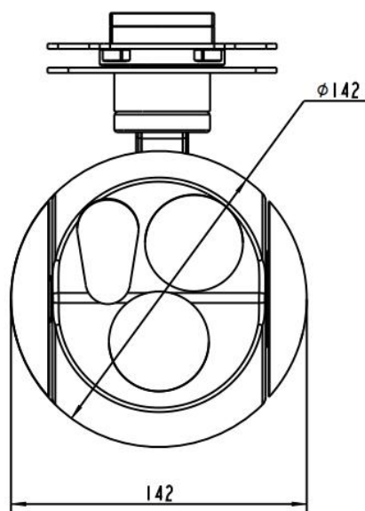
图 1-1-1 三光一体云台结构
