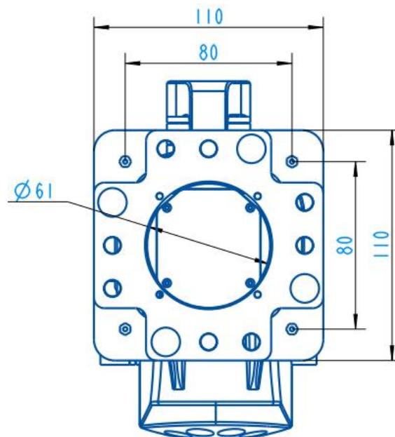
图 3-1-1：双光云台对外机械接口
