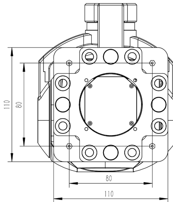
图 3-1-1：双光云台对外机械接口
