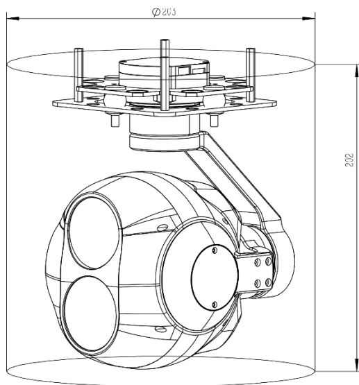
图 1-1-1 双光一体云台结构
