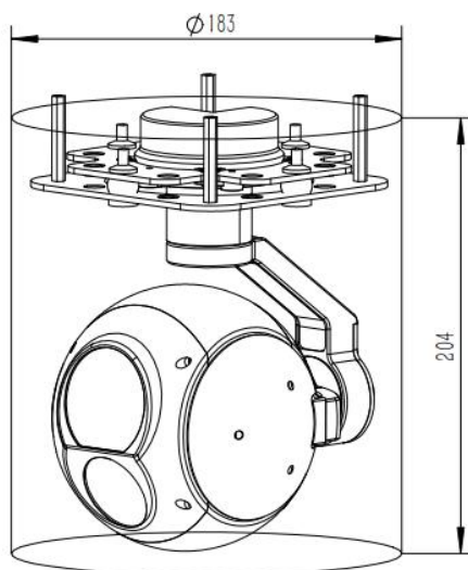
图 1-1-1 云台结构
