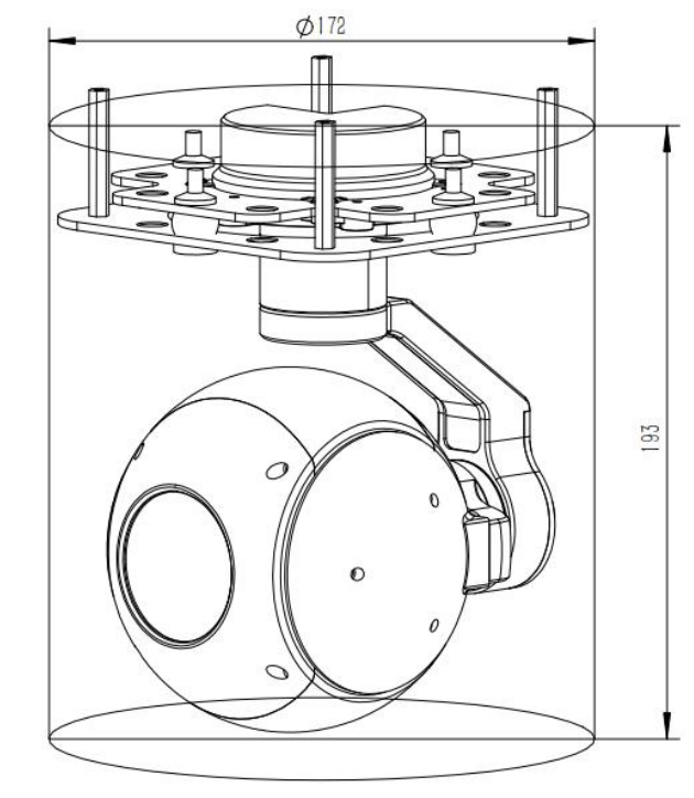
图 1-1-1 云台结构
