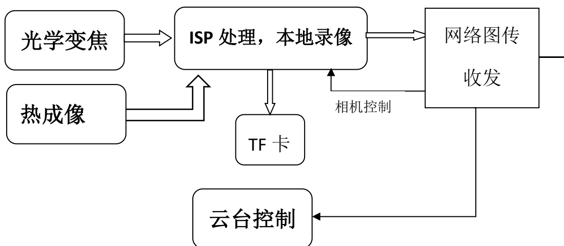
图 1-2-1 系统功能框架
